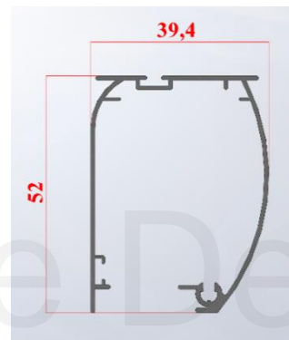
Kaseta.
