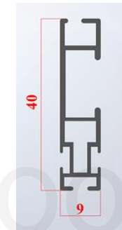
Donji profil.
