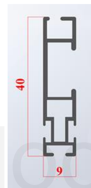
Donji profil.
