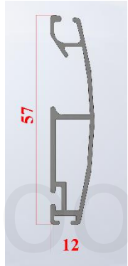
Donji profil.
