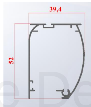
Kaseta.
