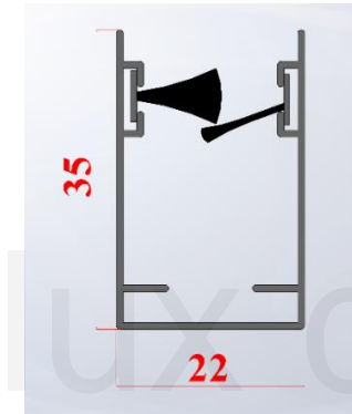
Vodilica.
