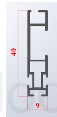
Donji profil.
