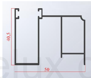
Vodilica.
